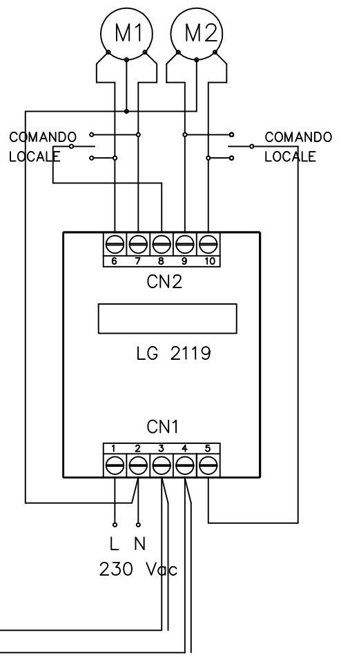
COMANDO 2 MOTORI CON PROTEZIONE VENTO
